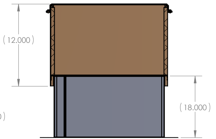
SECTION B-B SCALE 1 : 16
